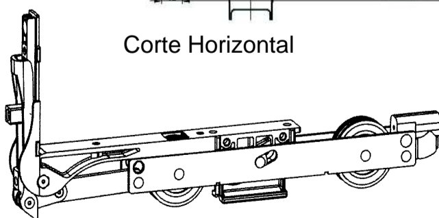
Carro dianteiro
