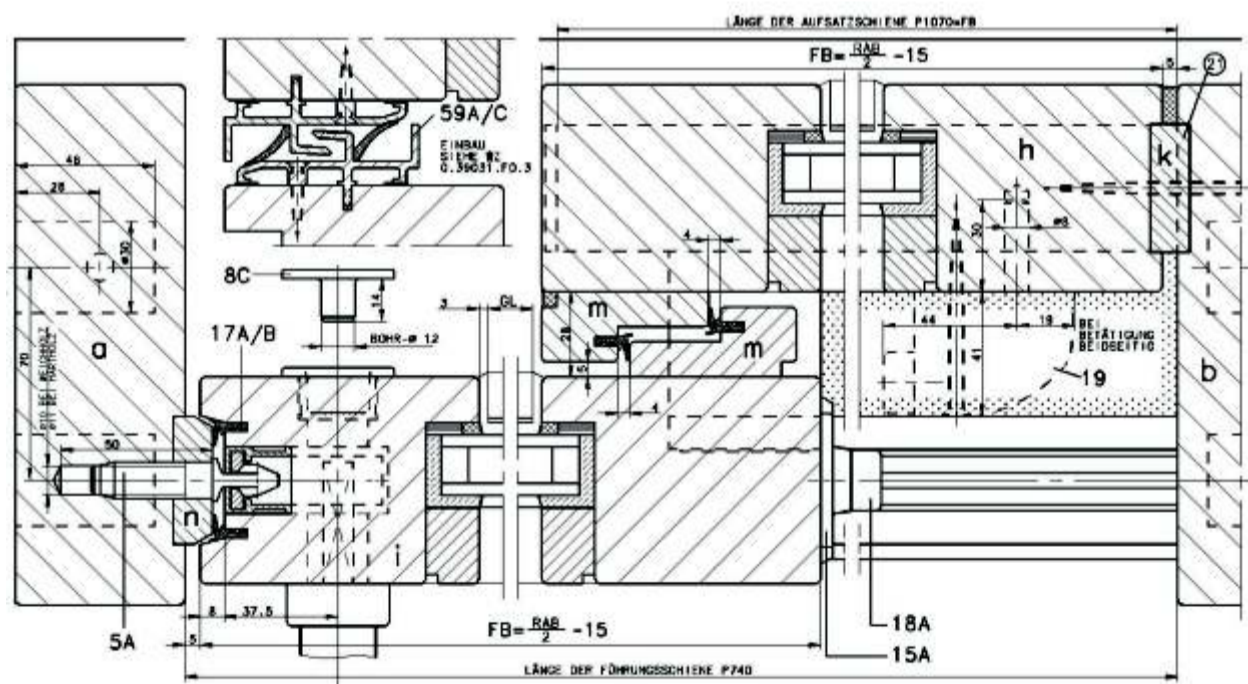
Corte Horizontal
